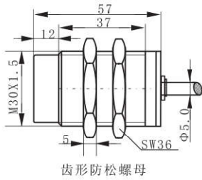
齿形防松螺母
